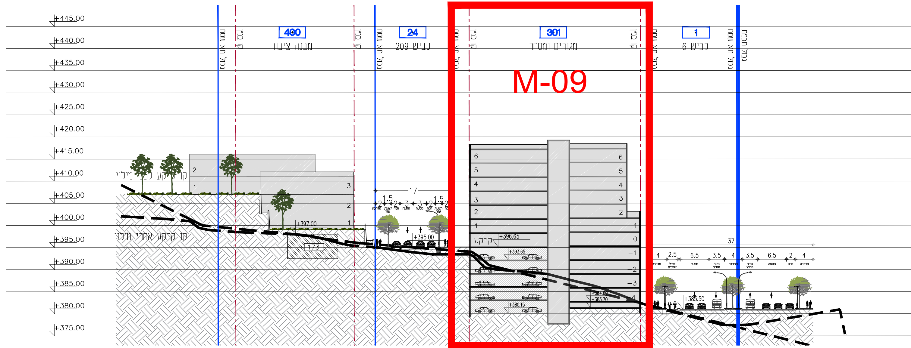
חתך 17-17
