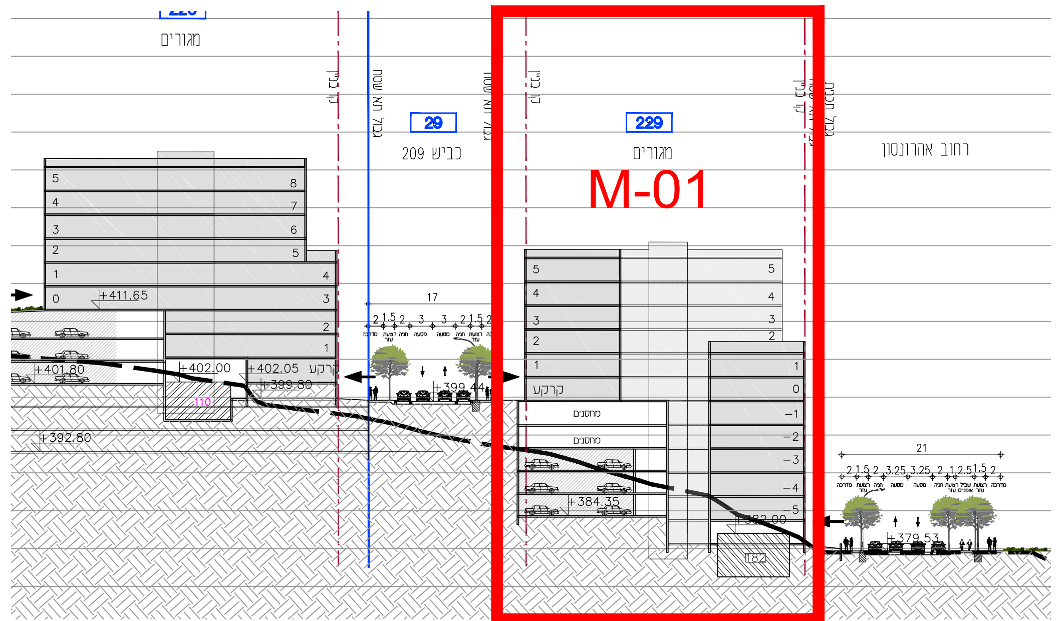
חתך C-C
