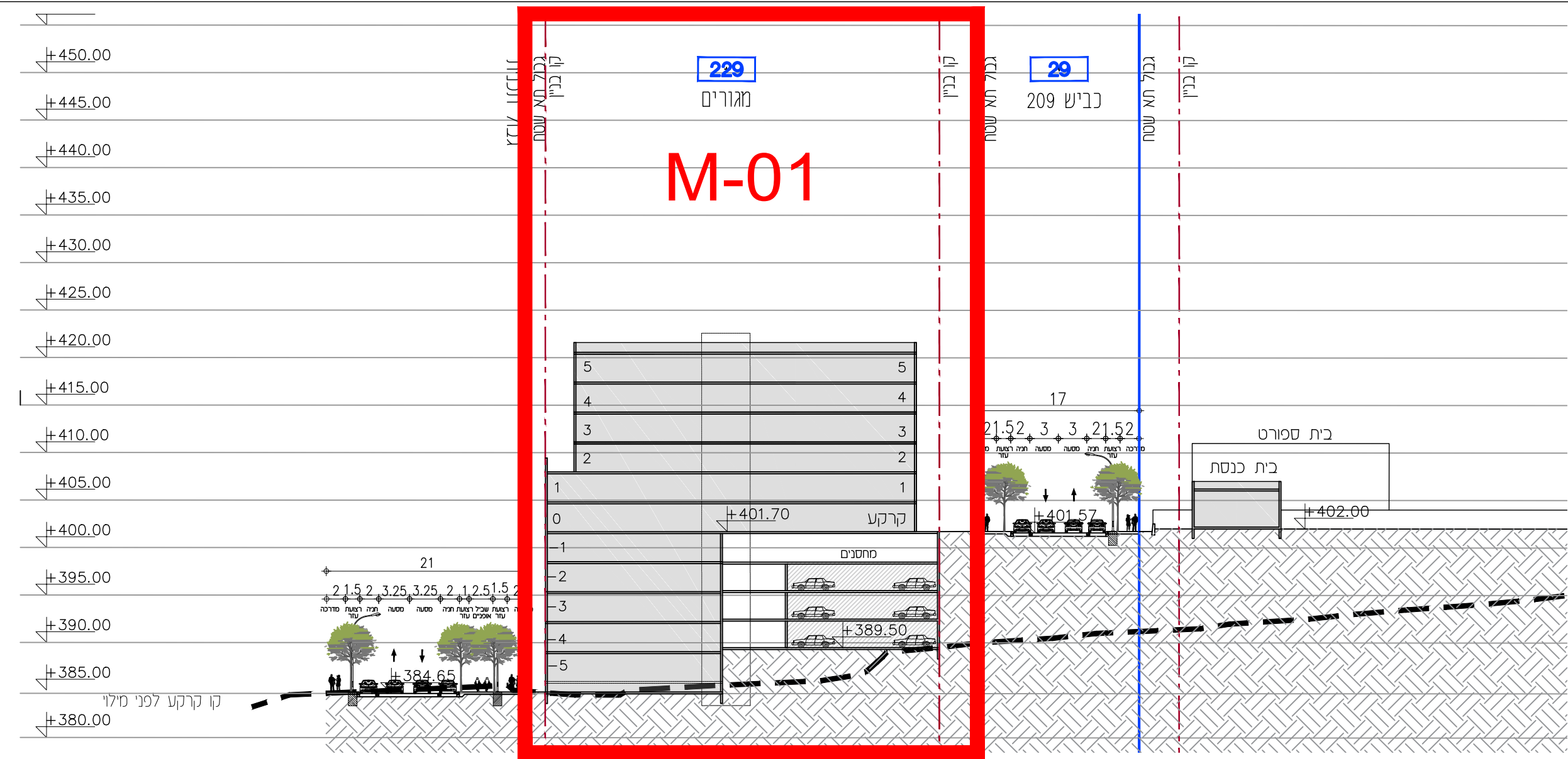
חתך A-A
