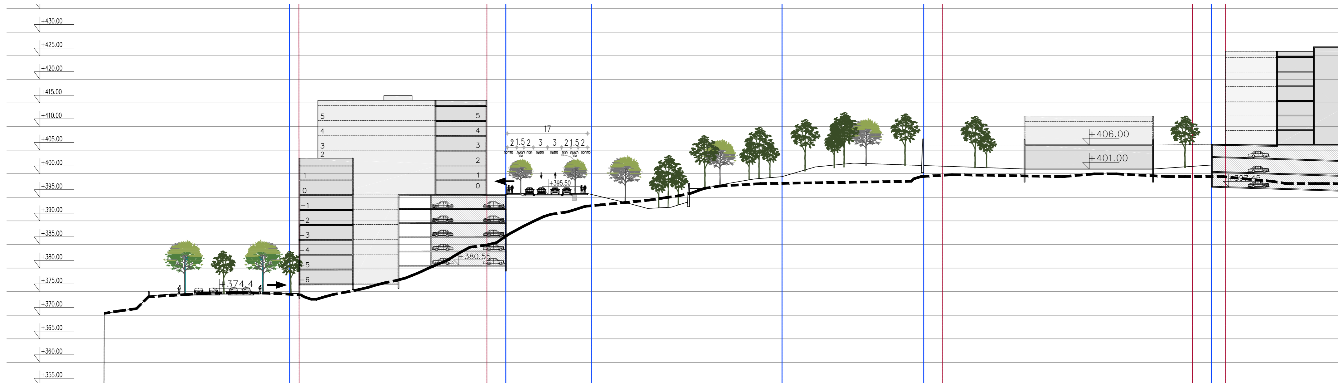
חתך E-E
