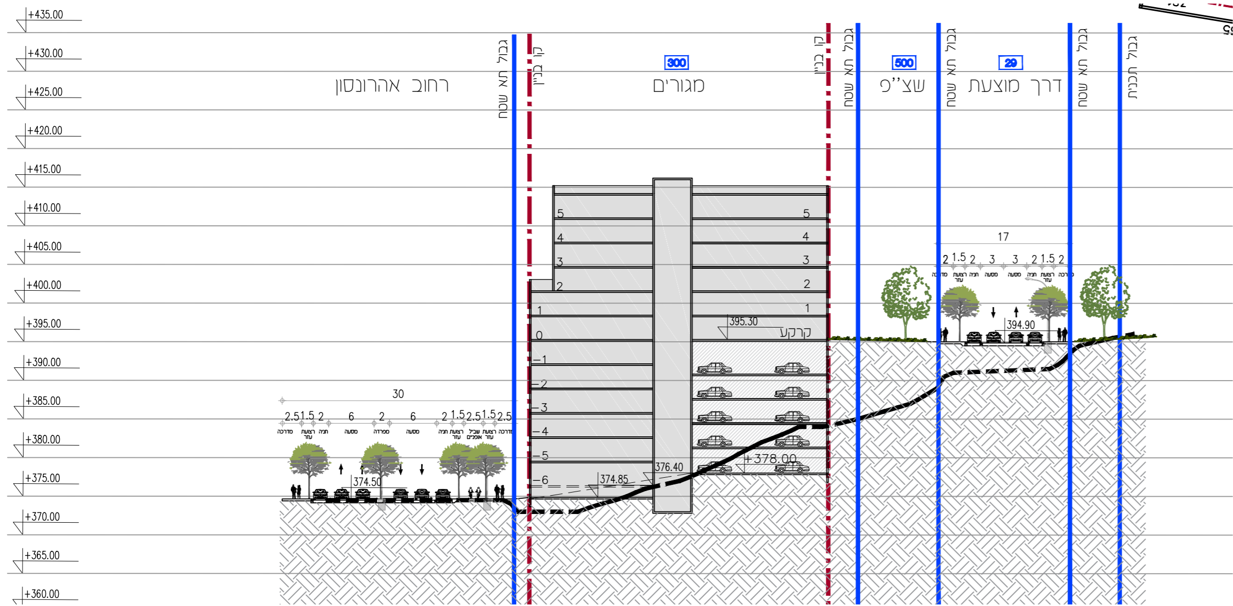
חתך F-F
