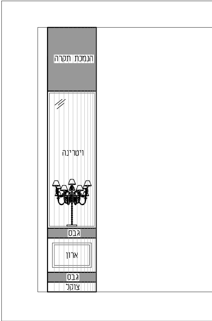
חזית
