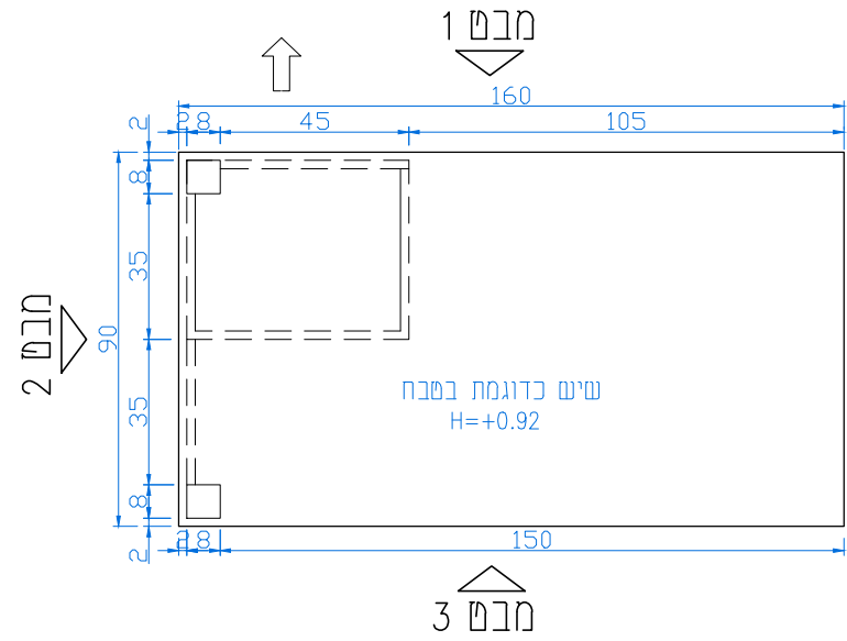
תכנית אי קני"מ 1-20
