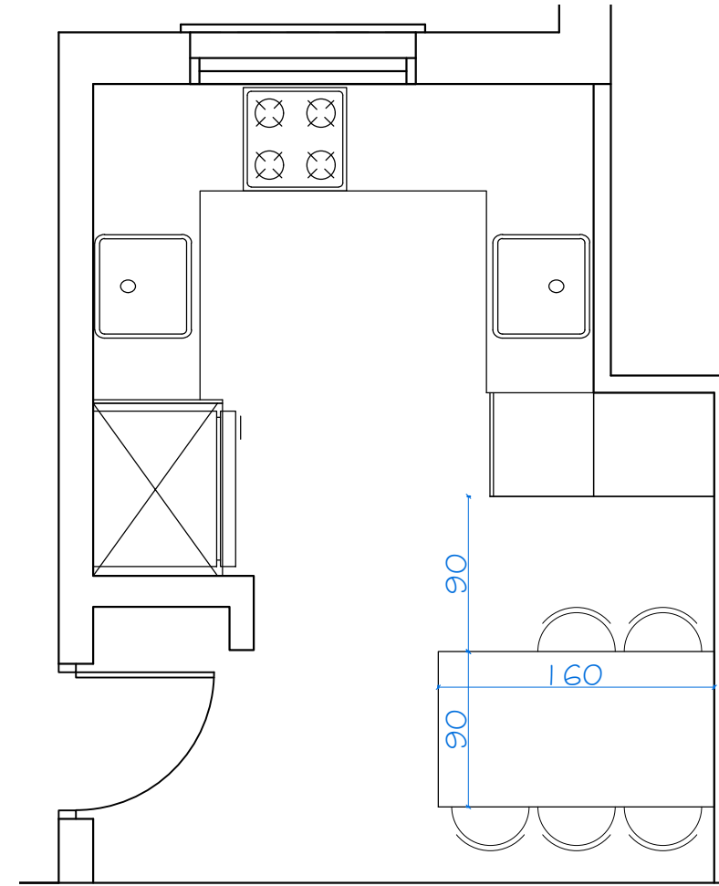
תכנית מטבח קני"מ 1-50
