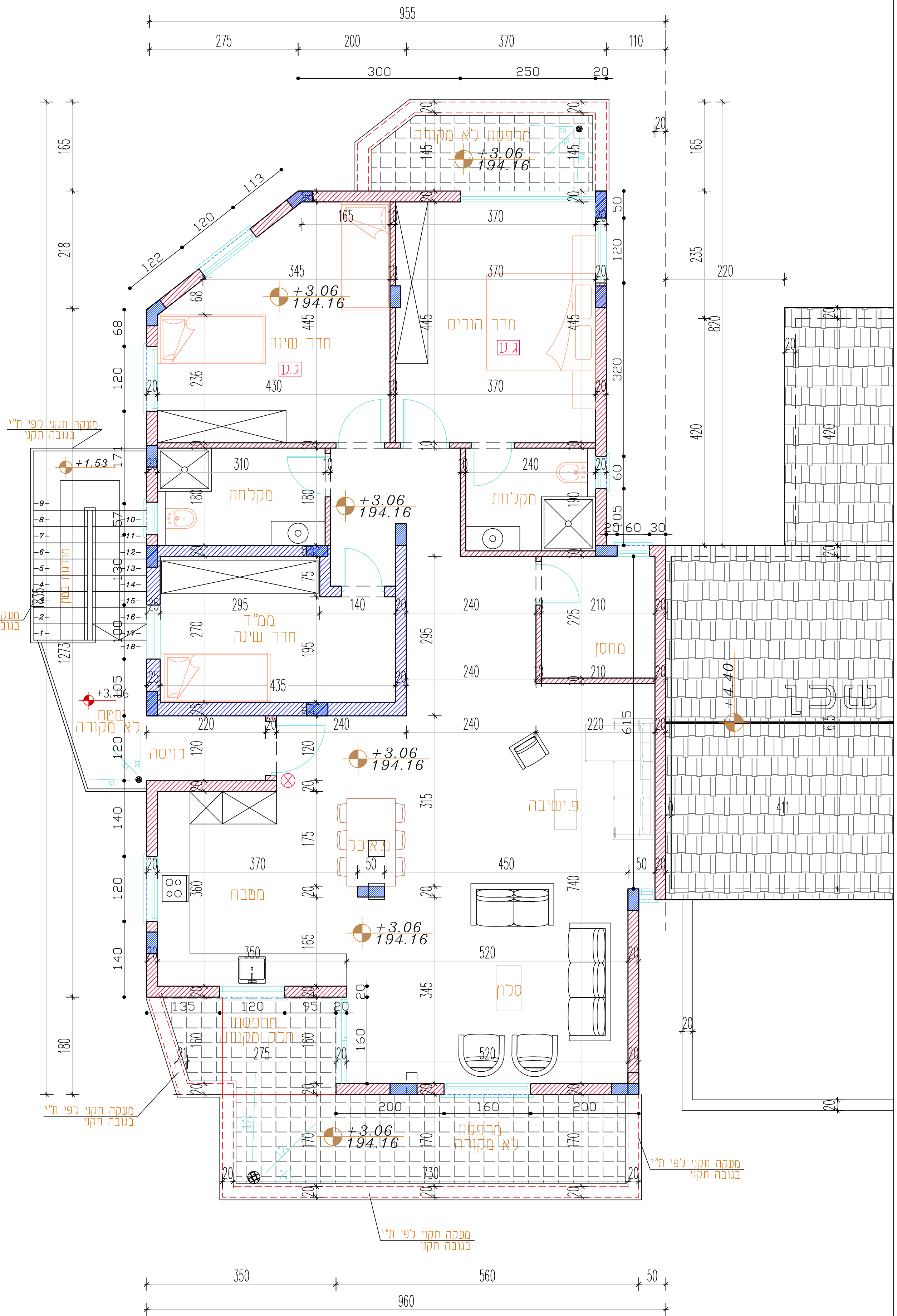
תכנית קומה -א- קנ"מ 1:50
