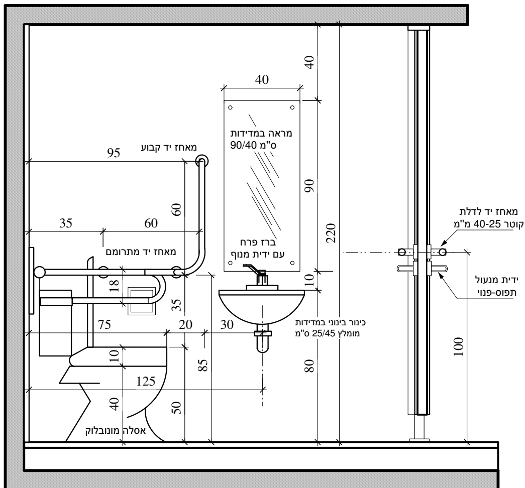
חזית קנ"מ 1:20
