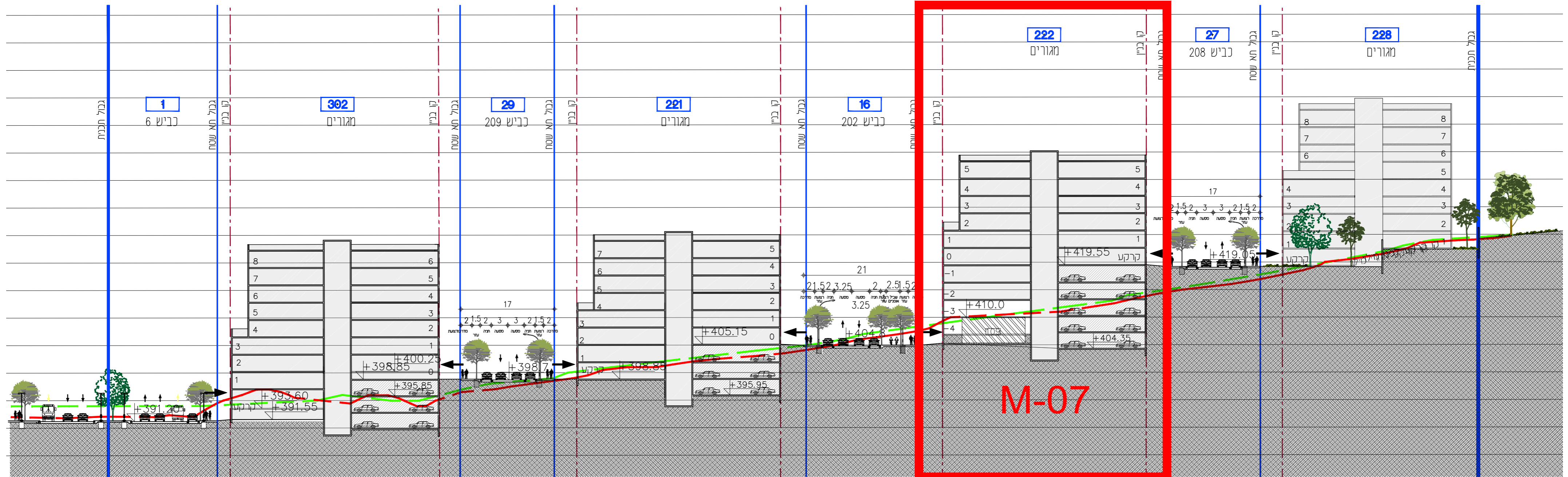
חתך 15-15
