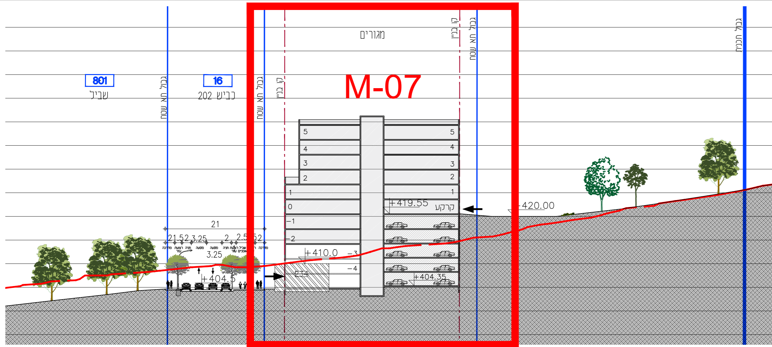
חתך M7-M7
